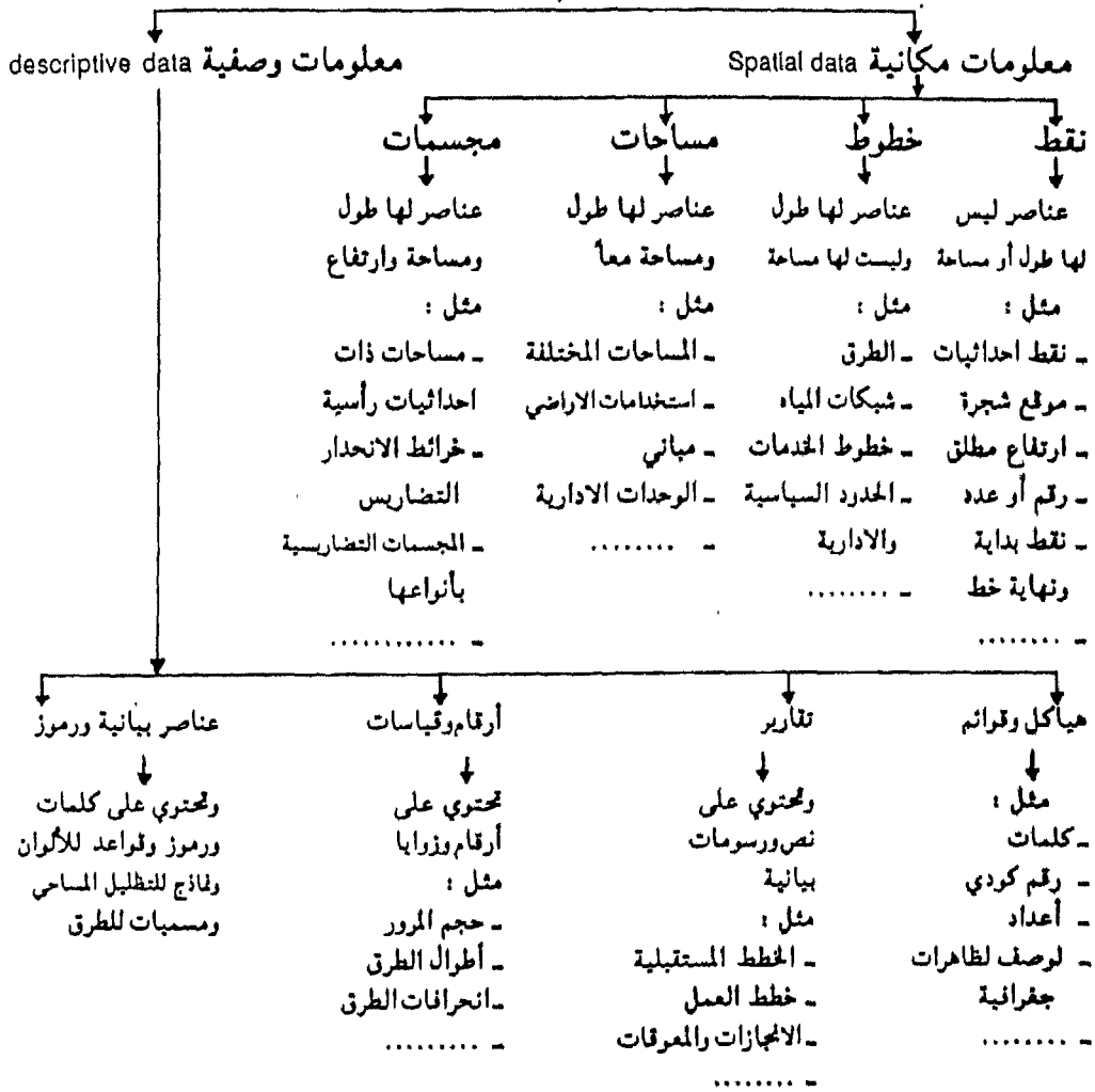
شكل (١٤) : يوضح المكونات الأساسية لقاعدة المعلومات الجغرافية
